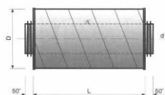
Rohrschalldämpfer mit Safe-Muffen Amortisseurs de bruit avec manchons Safe
